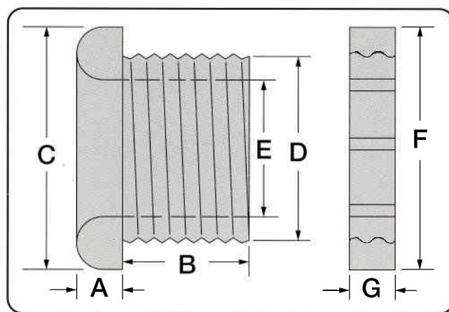
ブッシング寸法 (単位: mm)
